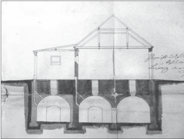
Bauzeichnung 1868 von Maurermeister Moritz Kornagel, das Anlegen eines dritten Kellers betreffend (Stadtarchiv Leipzig/StadtAL, BauA 23748 Bl. 11 – Auszug)
